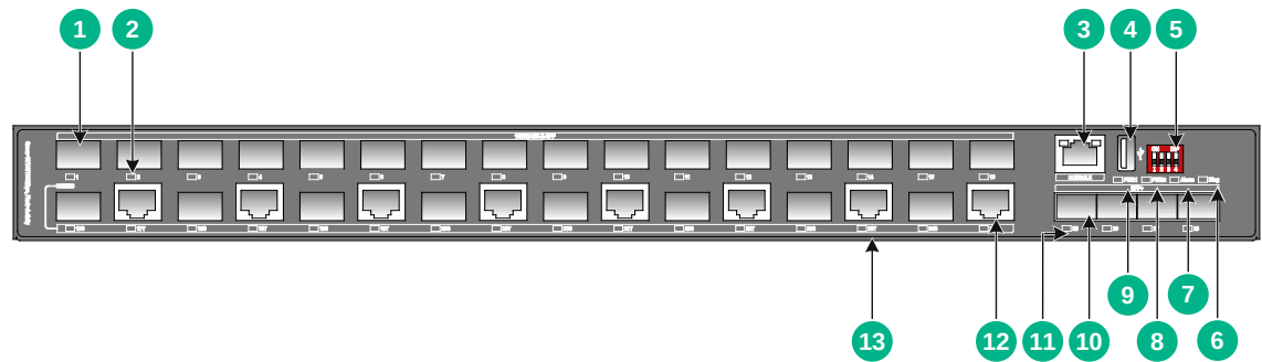
图2-3 IE4320-28F 前面板示意图
