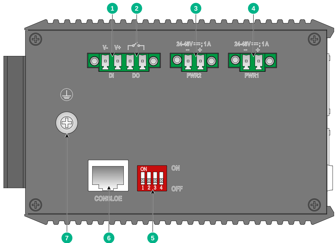
图2-2 IE4320-20P 上面板示意图
