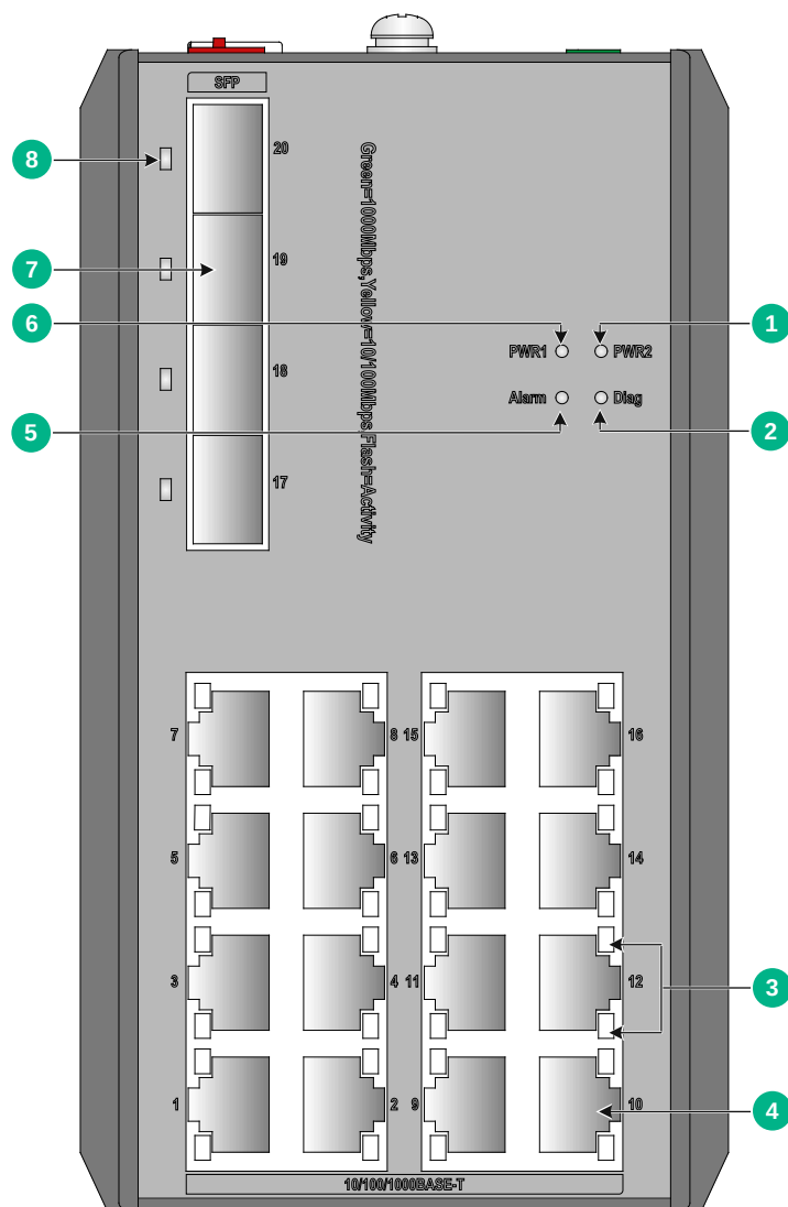
图2-1 IE4320-20P 前面板示意图
