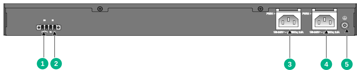
图2-4 IE4320-28F 后面板示意图
